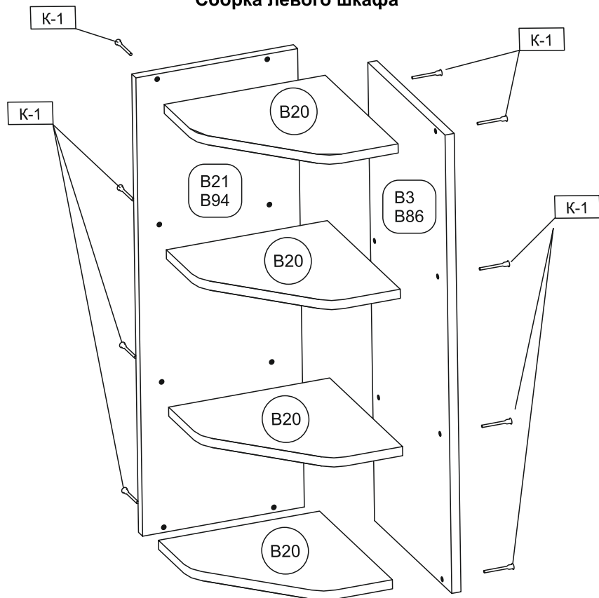
Сборка левого шкафа
