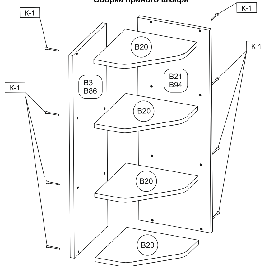
Сборка правого шкафа
